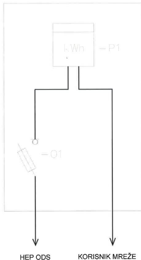
Slika 1. Kućni priključno mjerni ormar (KPMO) za 1 OMM - P \leq 50 \text{ kW} (izravno mjerenje)
